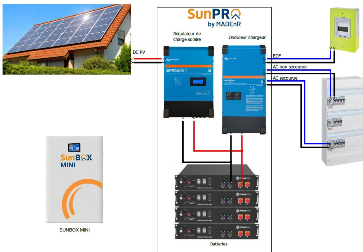
Figure 54 : Schéma de principe de la SunBox Mini
