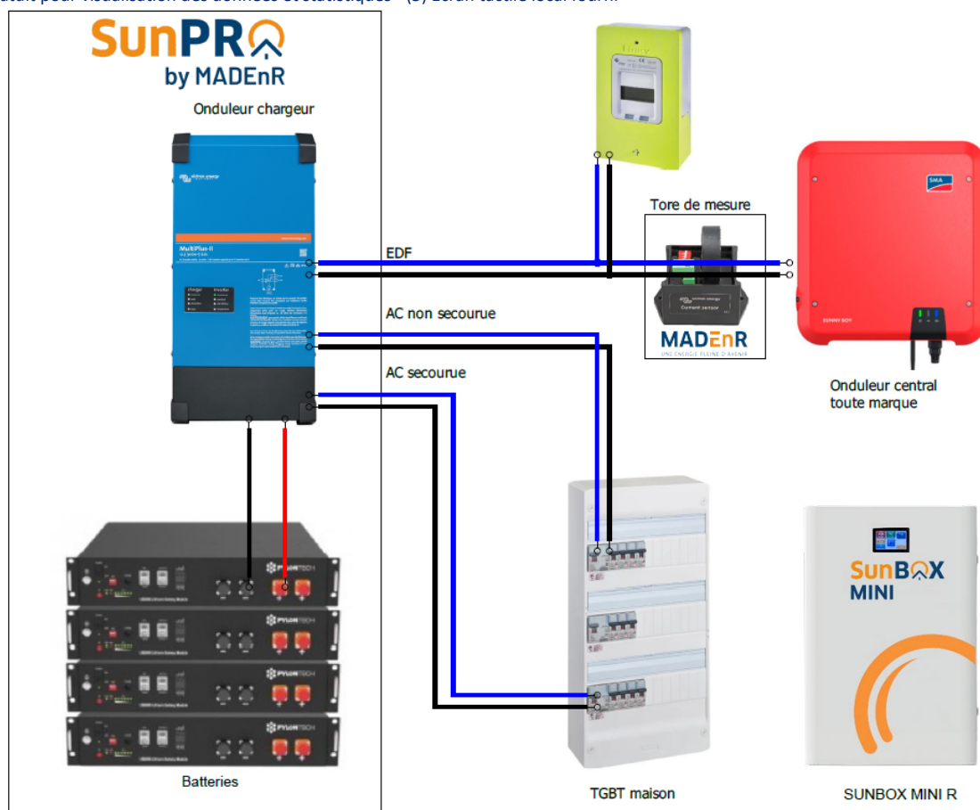
Figure 55 : Schéma de principe de la SunBox Mini R
