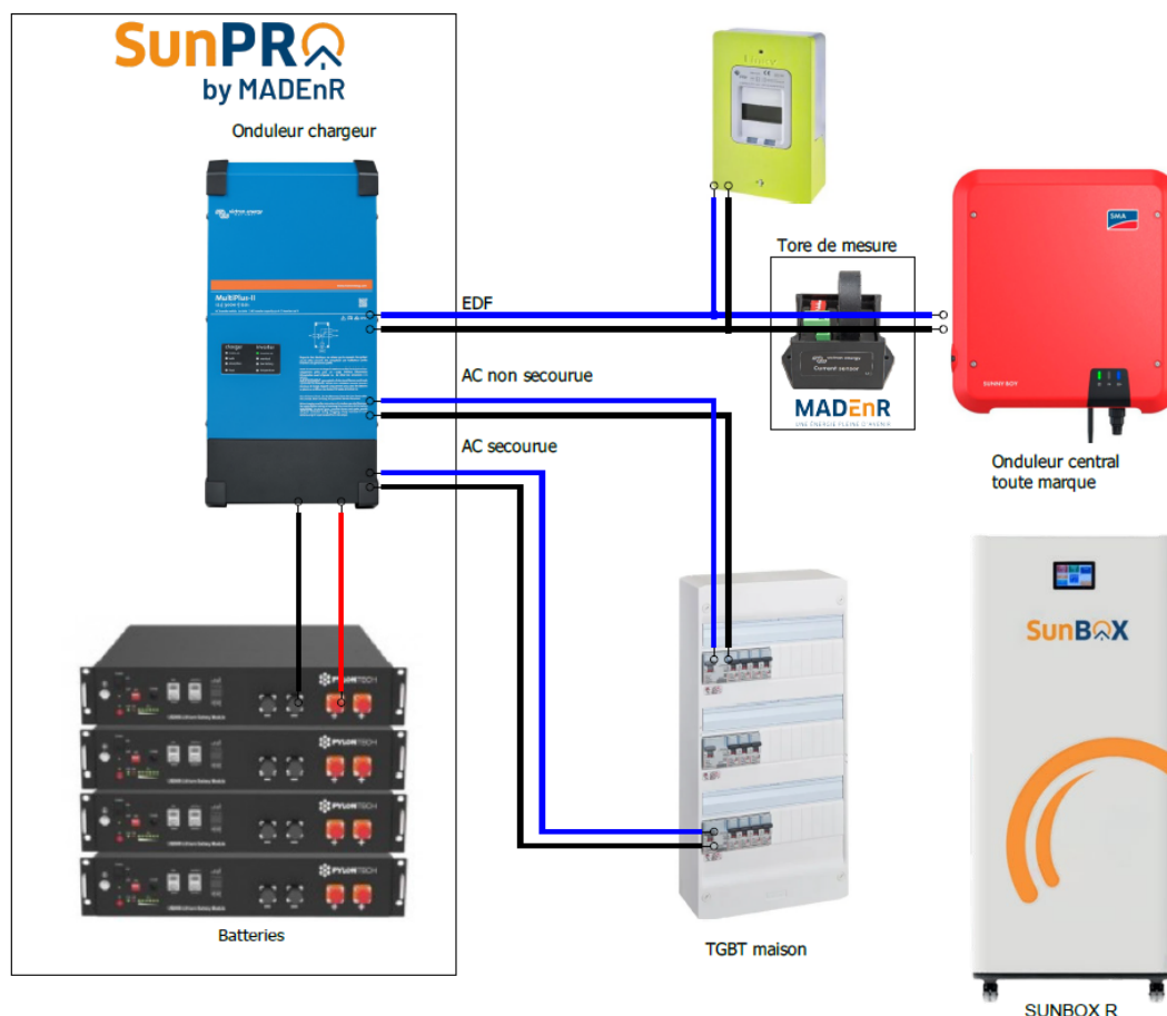
Figure 53 : Schéma de principe de la SunBox R
